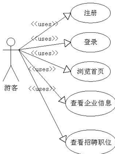
图 1-1 游客功能用例图
