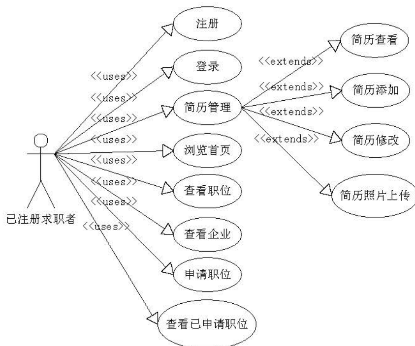
图 1-1 已注册求职者功能用例图
